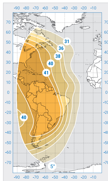
«Экспресс-АМ8», Фиксированный луч №2, С-диапазон Express-AM8 Fixed Beam No. 2, C band
