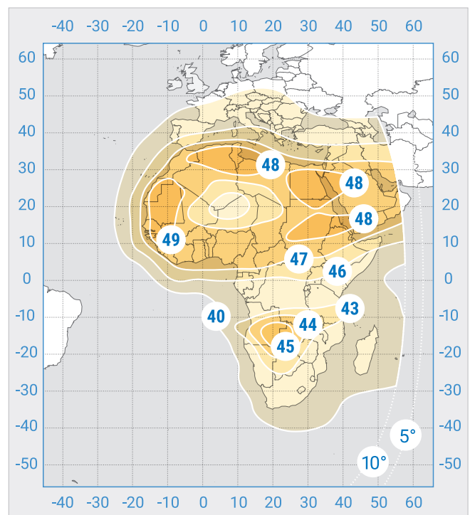
«Экспресс-AM8», Фиксированный луч №2, Ку-диапазон Express-AM8 Fixed Beam No. 2, Ku band
