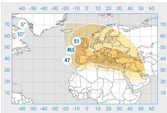
«Экспресс-AM8», Фиксированный луч №1, Ку-диапазон Express-AM8 Fixed Beam No. 1, Ku band
