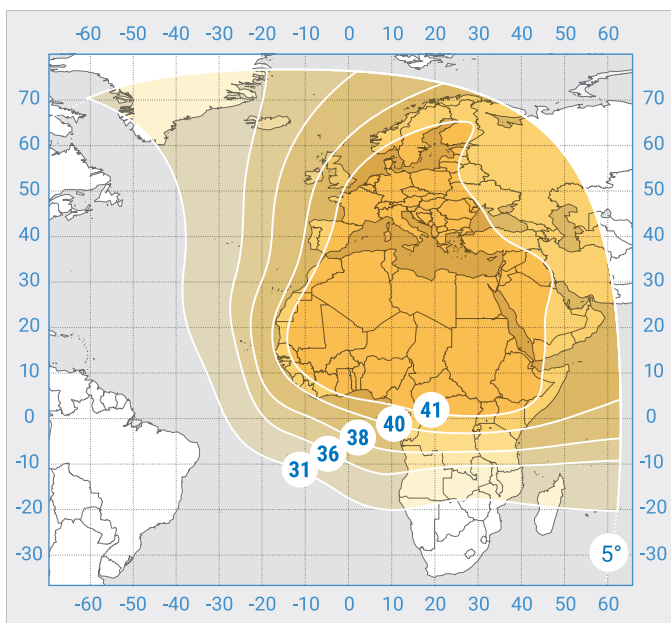
«Экспресс-АМ8», Фиксированный луч №1, С-диапазон Express-AM8 Fixed Beam No. 1, C band
